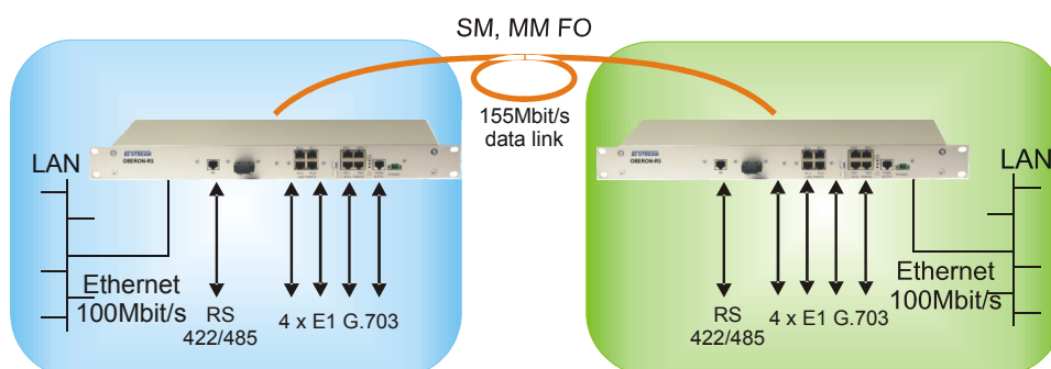
Rys. 1. Podstawowa konfiguracja pracy urządzenia OBERON-RS
